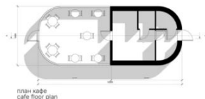
план кафе cafe floor plan
